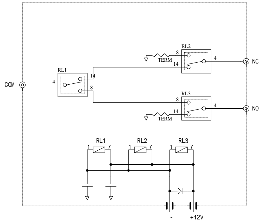
終端ありタイプ AV201, AV203, AV205, AV207
