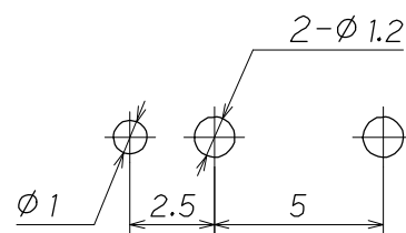
取付穴参考寸法
